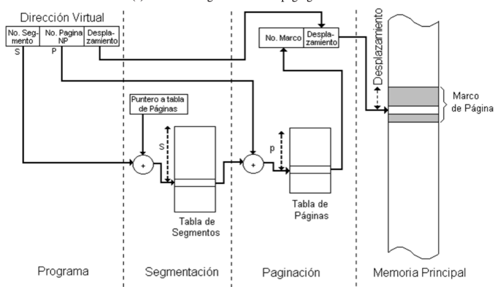
Traducción de dirección en la Segmentación Paginada.
